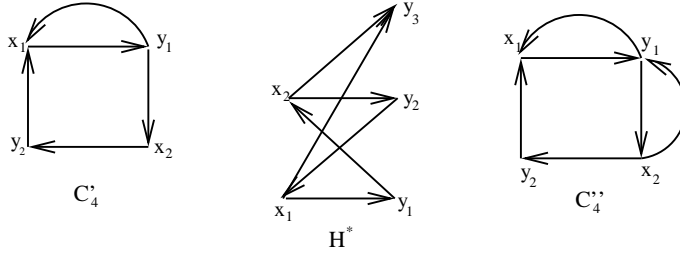
FIG. 1.2. The digraphs C'_4 , C''_4 and H^*
